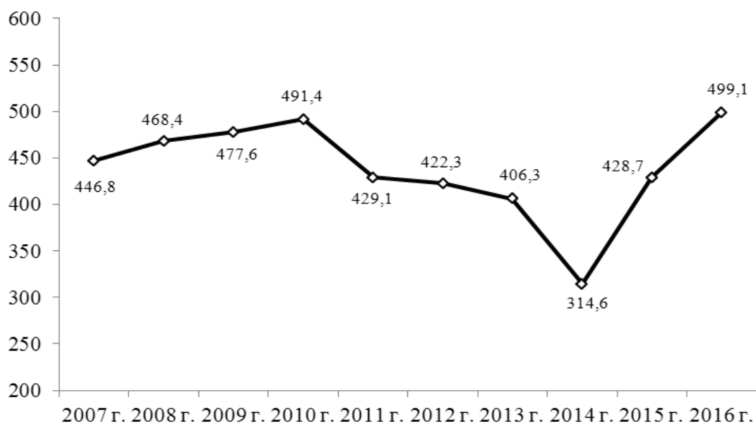
Рис. 5. Коллективные дозы медицинского облучения населения Республики Карелия, 2007-2016 г.г., чел.-Зв в год
