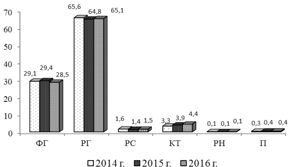
Рис. 4. Доля различных видов рентгенорадиологических процедур, проведённых в Республике Карелия, 2014 – 2016 г.г., %
